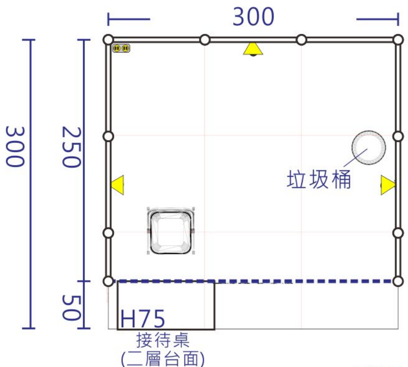
平面圖
